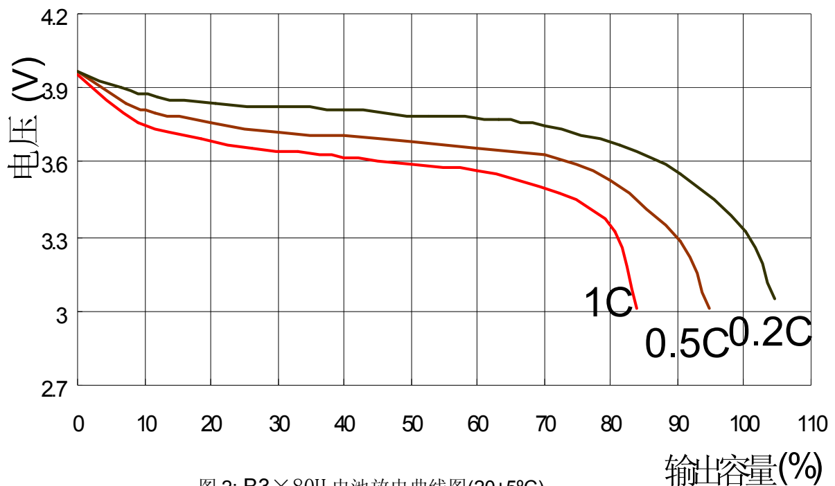
图 2: B3×80H 电池放电曲线图(20±5°C)
