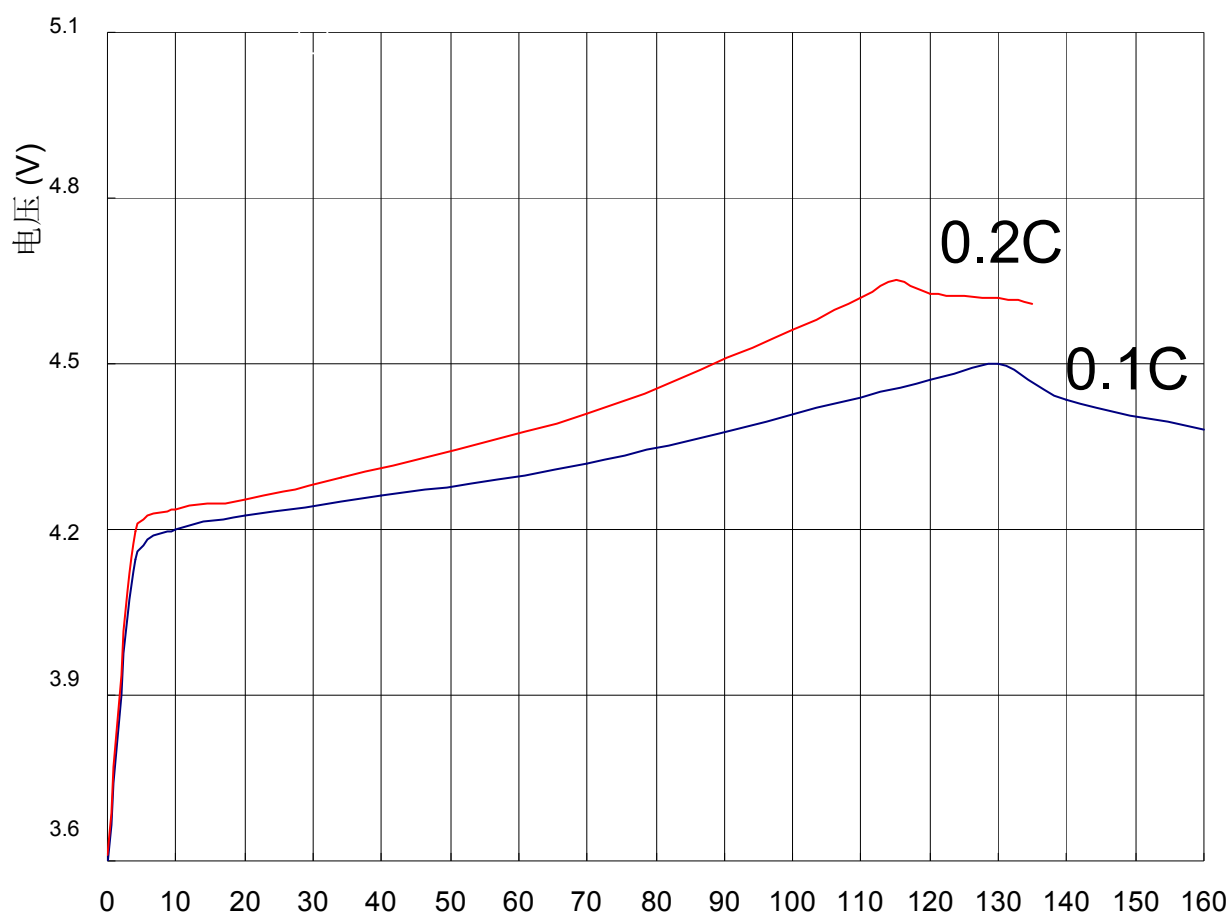
图 1: B3×80H 电池充电曲线图(20±5°C)
