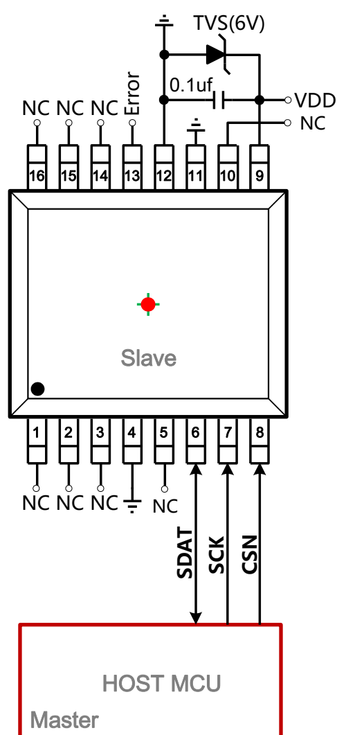
图-15：3线SPI参考电路
