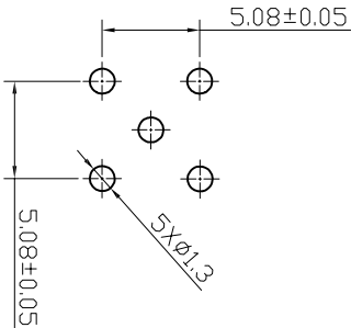
建议PCB印刷尺寸
