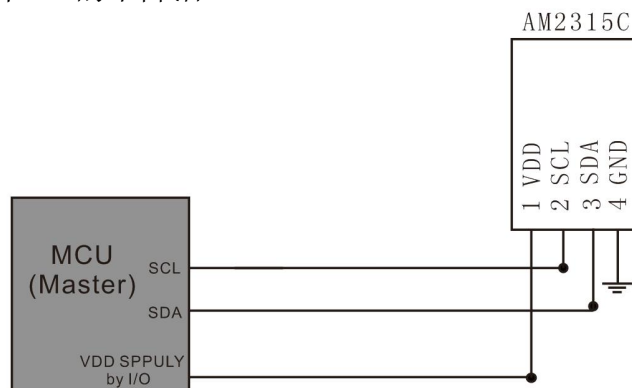
图8. 典型的应用电路
