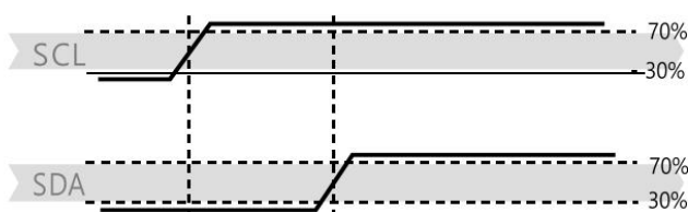
图 11. 停止传输状态 (P) - 当SCL高电平时, SDA线上从低电平转换为高电平。停止状态是由主机控制的一种特殊的总线状态,
