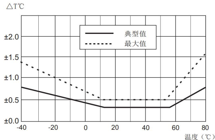
图3. 温度典型误差和最大误差 1
