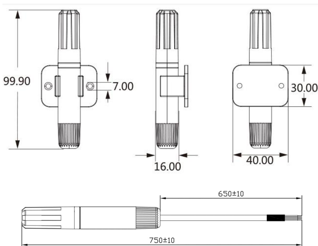
图12. AM2315C传感器封装图（单位：mm，未标明公差：±0.2mm）
