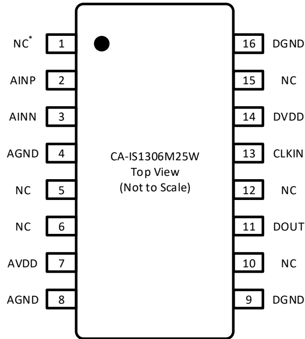
图 6-3 CA-IS1306M25W 引脚配置
