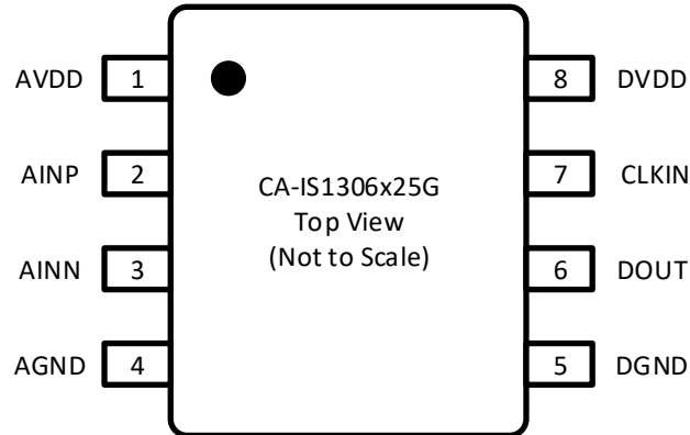
图 6-1 CA-IS1306x25G 引脚配置
