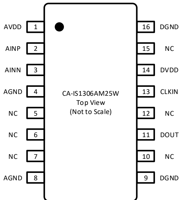
图 6-2 CA-IS1306AM25W 引脚配置
