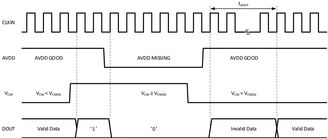
图 8-5 CA-IS1306x 安全故障输出波形
