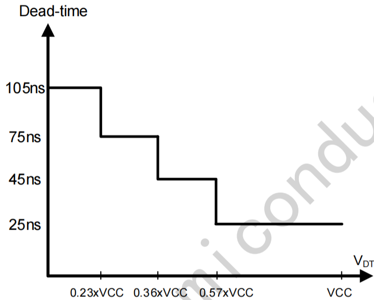
图 8-6 IRS2092S中死区时间与 V_{DT} 的关系
