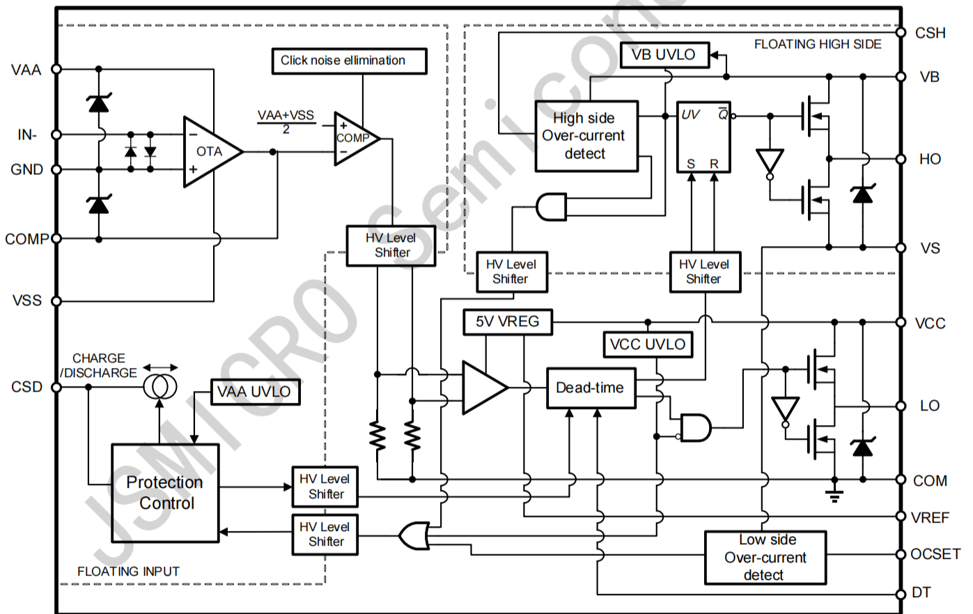
图 8-1 全芯片功能框图
