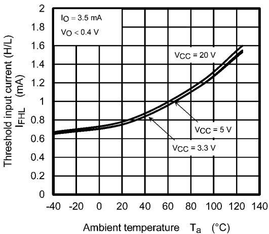
Fig. 12.2.11 I_{FHL} - T_a
