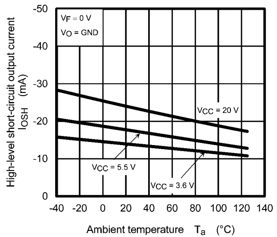
Fig. 12.2.10 I_{OSH} - T_a
