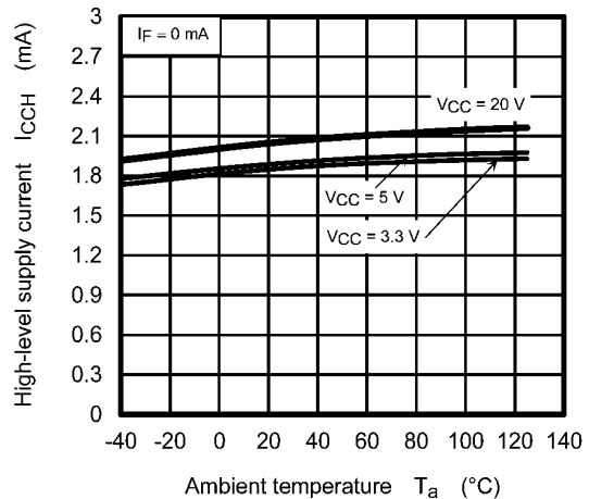
Fig. 12.2.8 I_{CCH} - T_a
